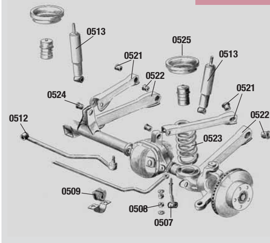
essieu avant XJ
