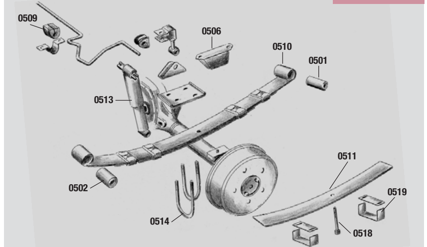
essieu arrière XJ
